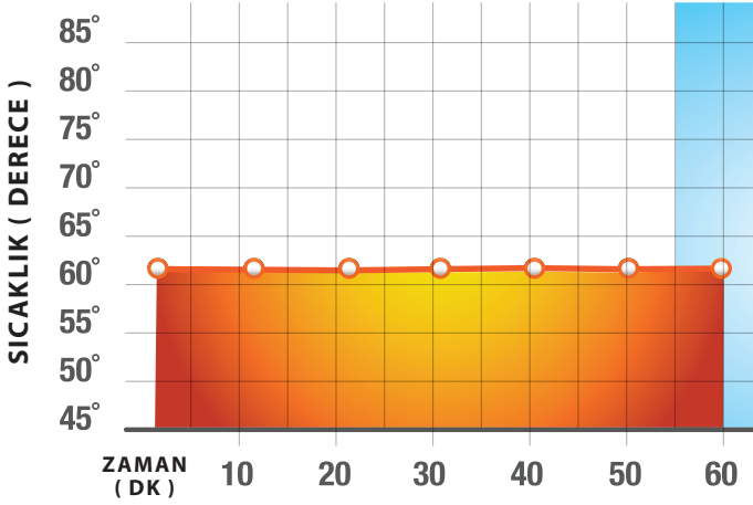
Camduction Sistemi Sıcaklık Muhafaza Sonuçları
